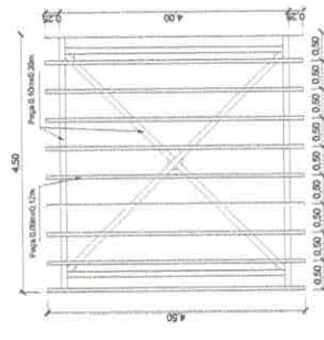
DETALHE DA ESTRUTURA DO ASSOALHO (ESC. 1:50)
