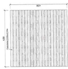
DETALHE DA ESTRUTURA DO ASSOALHO ESC. 1/25
