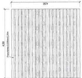
DETALHE DA DO ASSOALHO ESC: 1/20
