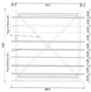
DETALHE DA ESTRUTURA DO ASSOALHO - ESC. 1/20
