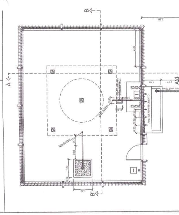
PLANTA BAIXA INSTALACOES AGUA FRIA Esc. 1:60
